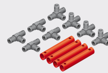
Bodenveranker bestehend aus Roh- ren und Kupplungen Ground anchoring consisting of pipes and connectors 1x
