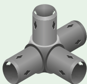
Raumkupplung 4-armig 4 way connector 14x 000 41
